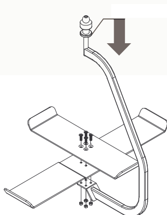
Рисунок 1.10 – Порядок сборки кронштейнов платформы
