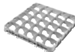
E5 = полноразмерная доп. секция с отделениями 1/2 глубины для низкопрофильных стеклоизделий на ножке
