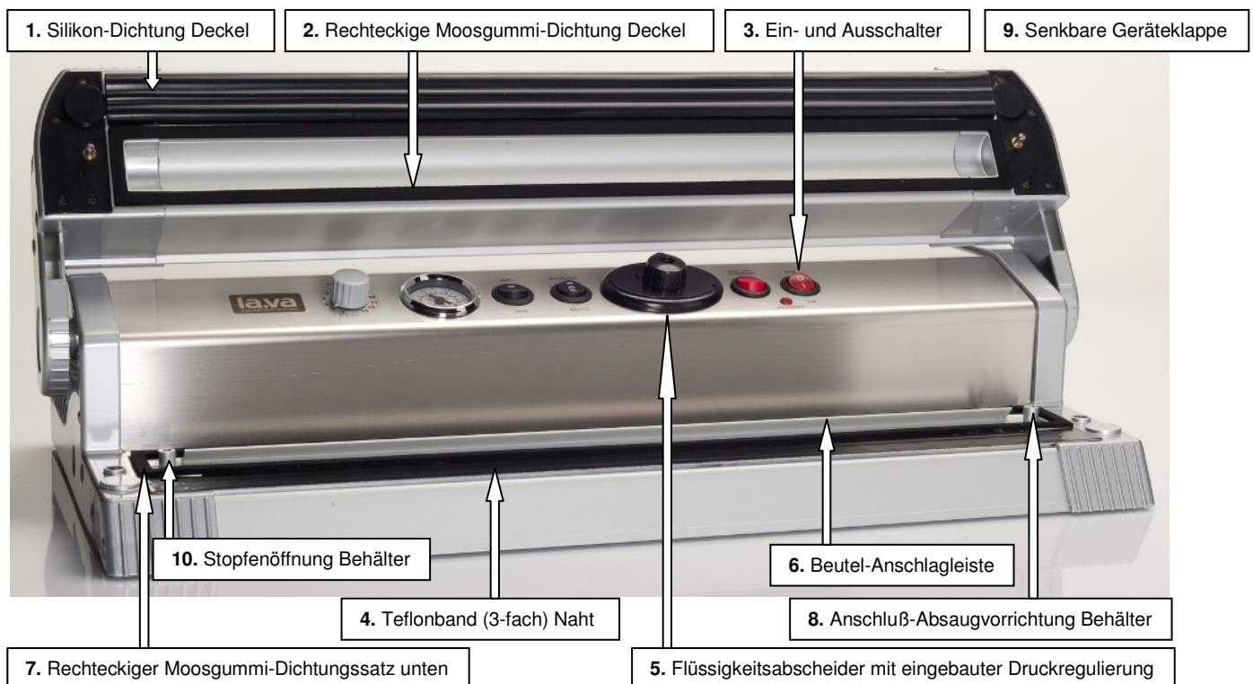
ABBILDUNG 1: Hauptbestandteile des V.350 ® Premium / V.400 ® Premium / V.500 ® Premium
