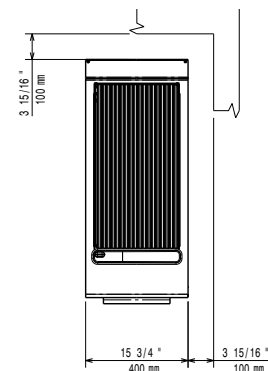
Вид сверху
