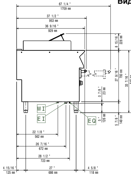
Вид сбоку
