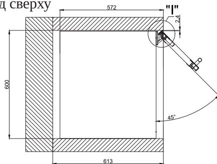
Вид сверху
