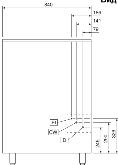
Вид спереди
