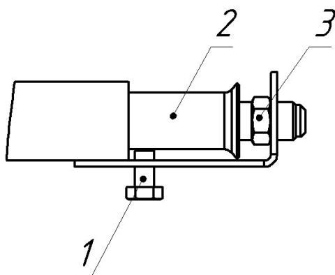
Рис. 2 Горелка духовки
