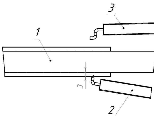
Рис. 3 Расположение электродов
