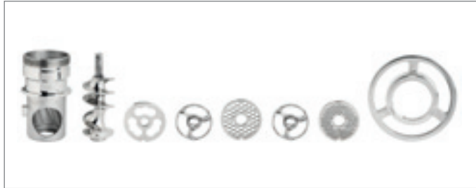
OPTIONAL: Bocca UNGER totale con 3 piastre e 2 coltelli Total UNGER mouth equipped with nr 3 plates and 2 knives
