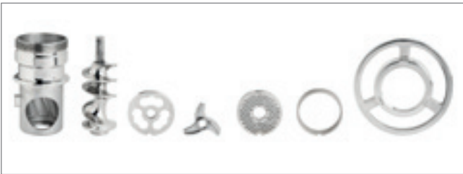
OPTIONAL: Bocca UNGER parziale con 2 piastre e 1 coltello Partial UNGER mouth equipped with nr 2 plates and 1 knife
