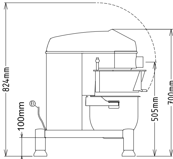
Вид сбоку
