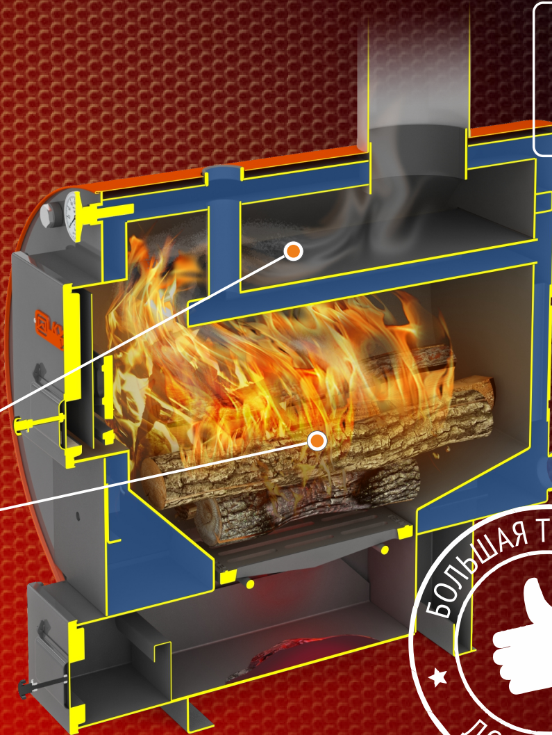
Котел в разрезе Куппер Уют
