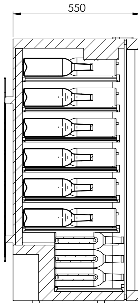
SECCIÓN B-B ESCALA 1 : 10
