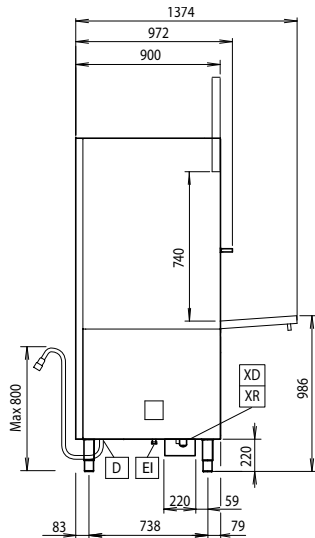
Вид сбоку
