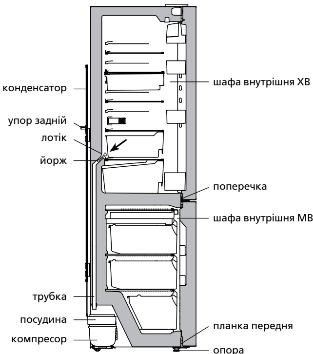
Малюнок 9 – Схема сливу талої води з ХВ
