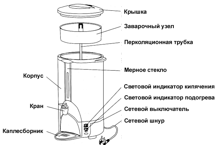
Рис.1. Основные узлы оборудования
