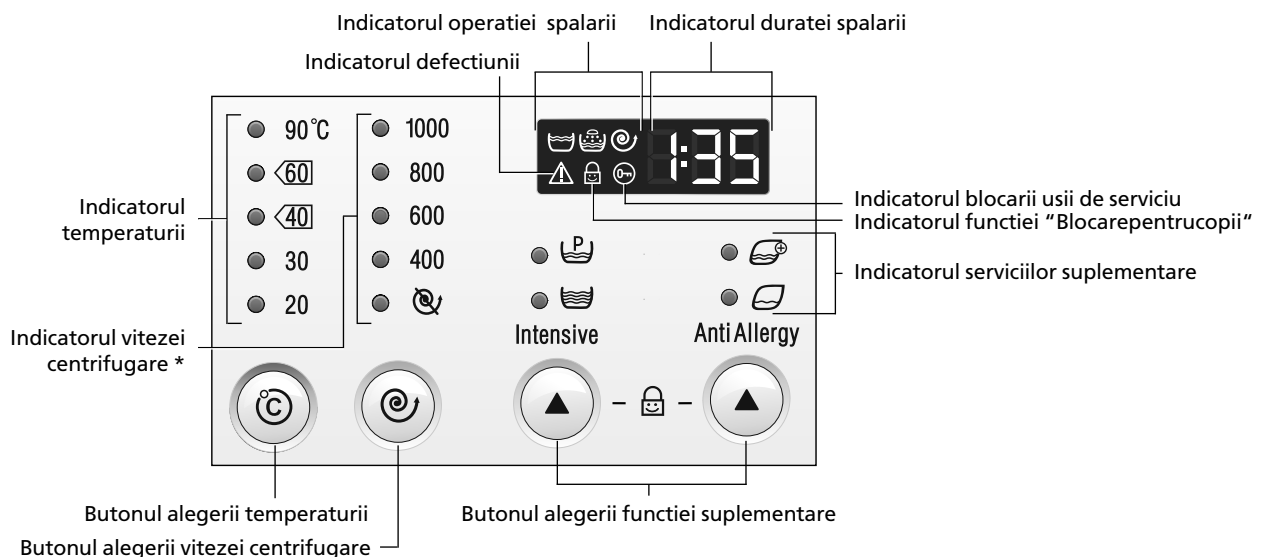
Figura 3 — Zona de indicare si butoanele alegerei functiilor suplimentare
