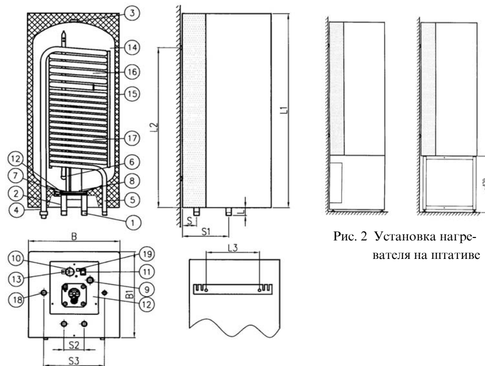
Рис. 1 Конструкция нагревателя
