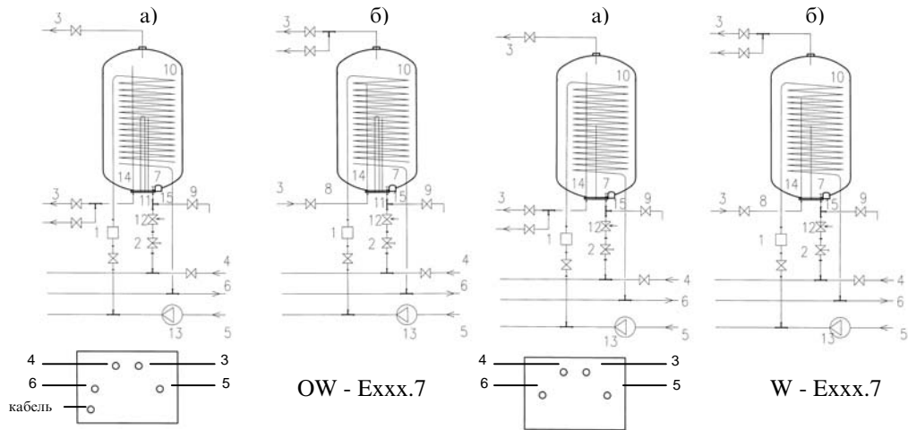
Рис. 5. Схема гидросистемы а) без циркуляции, б) с циркуляцией
