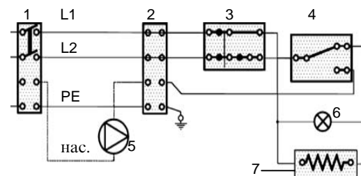
Рис. 3 Электросхема
