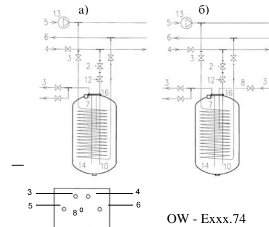
Рис. 5. Схема гидросистемы а) без циркуляции, б) с циркуляцией
