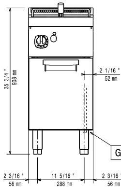
Вид спереди
