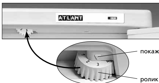
Рисунок 3 – Регулювання температури
